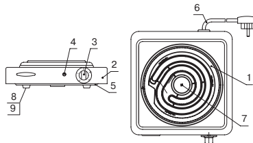
Рисунок 1 — Модель 114Т
